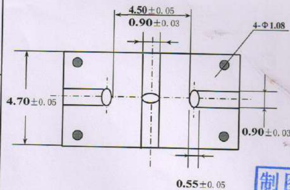
B-B' 斷面
