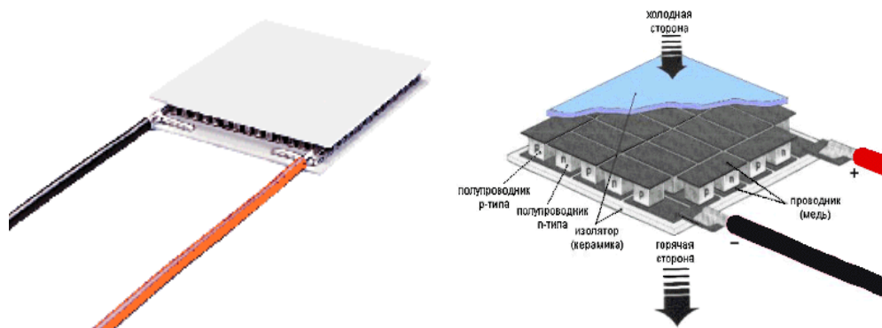
Рис.2 Так выглядят модули Пельтье.
