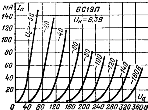
Анодные характеристики.
